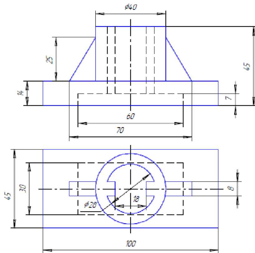
Рисунок 1 – Стойка
