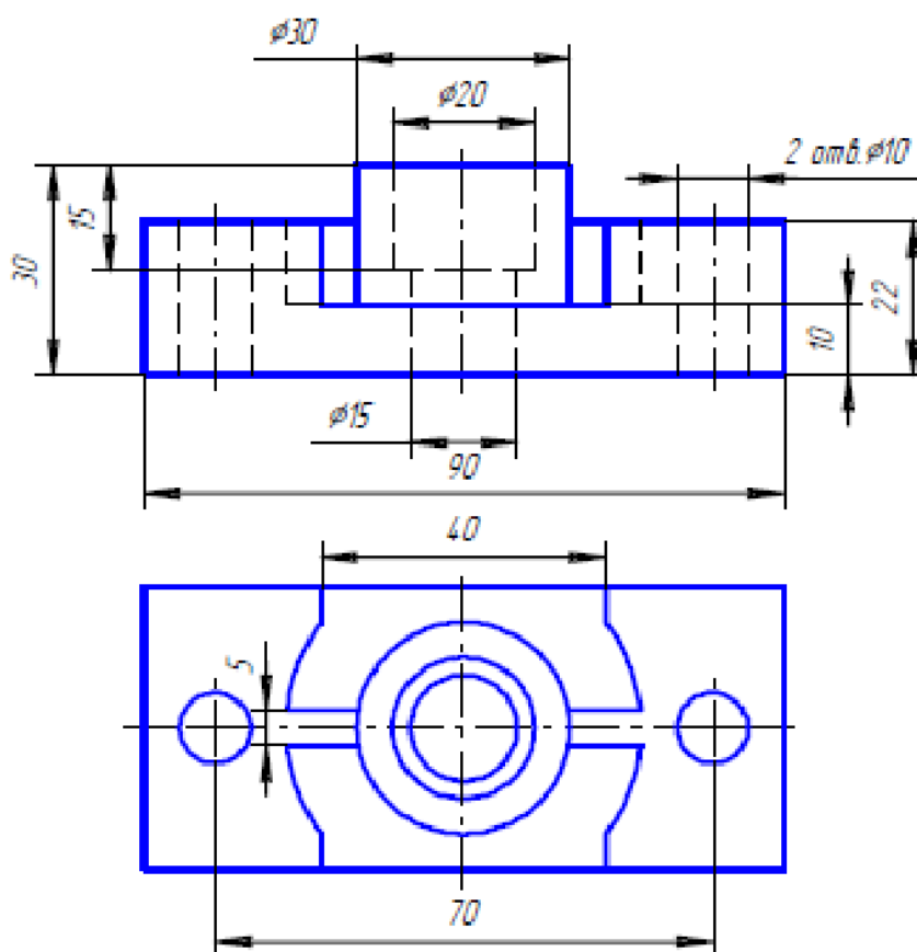
Рисунок 1 – Корпус
