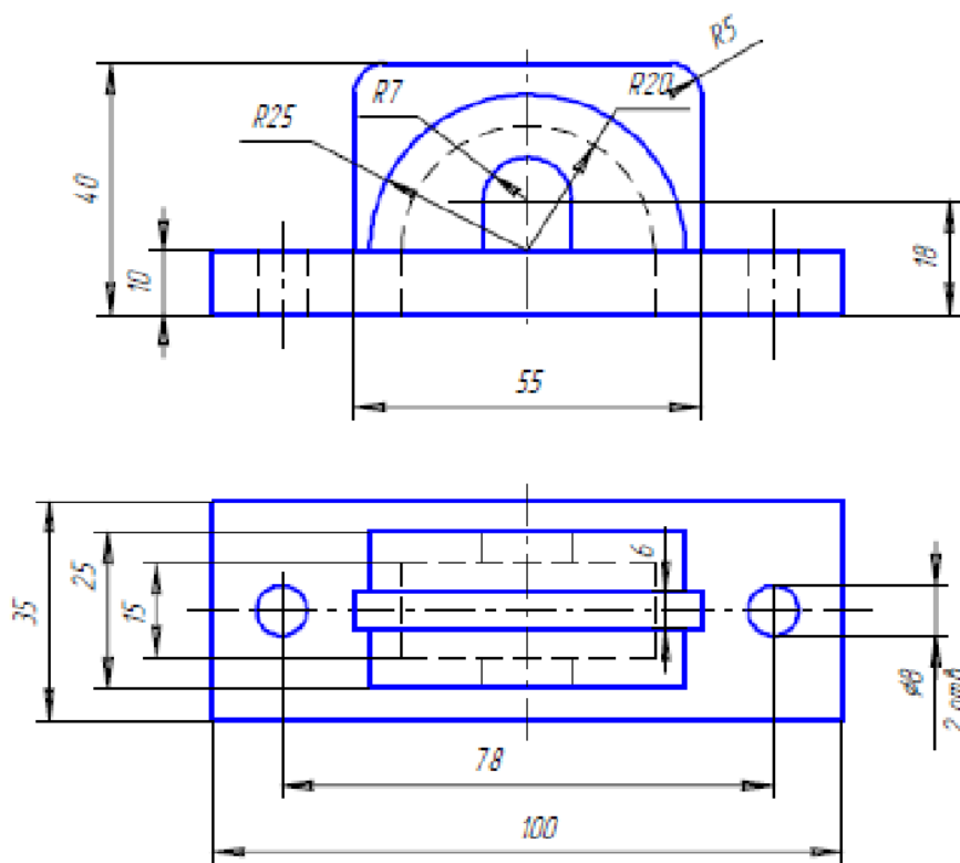
Рисунок 1 – Крышка
