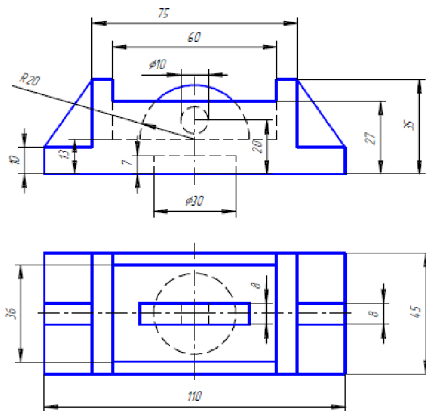
Рисунок 1 – Опора
